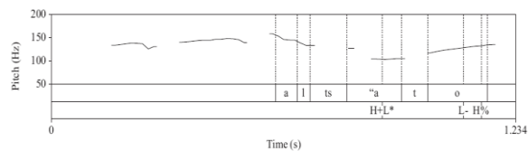
Fig.2 Interrogativa sì/no con DD prodotta da un parlante genovese: "C'ha il pollice alzato?"
