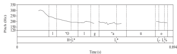
Fig.1 Dichiarativa con DD prodotta da una parlante genovese: "Ce l'ho il gatto".
