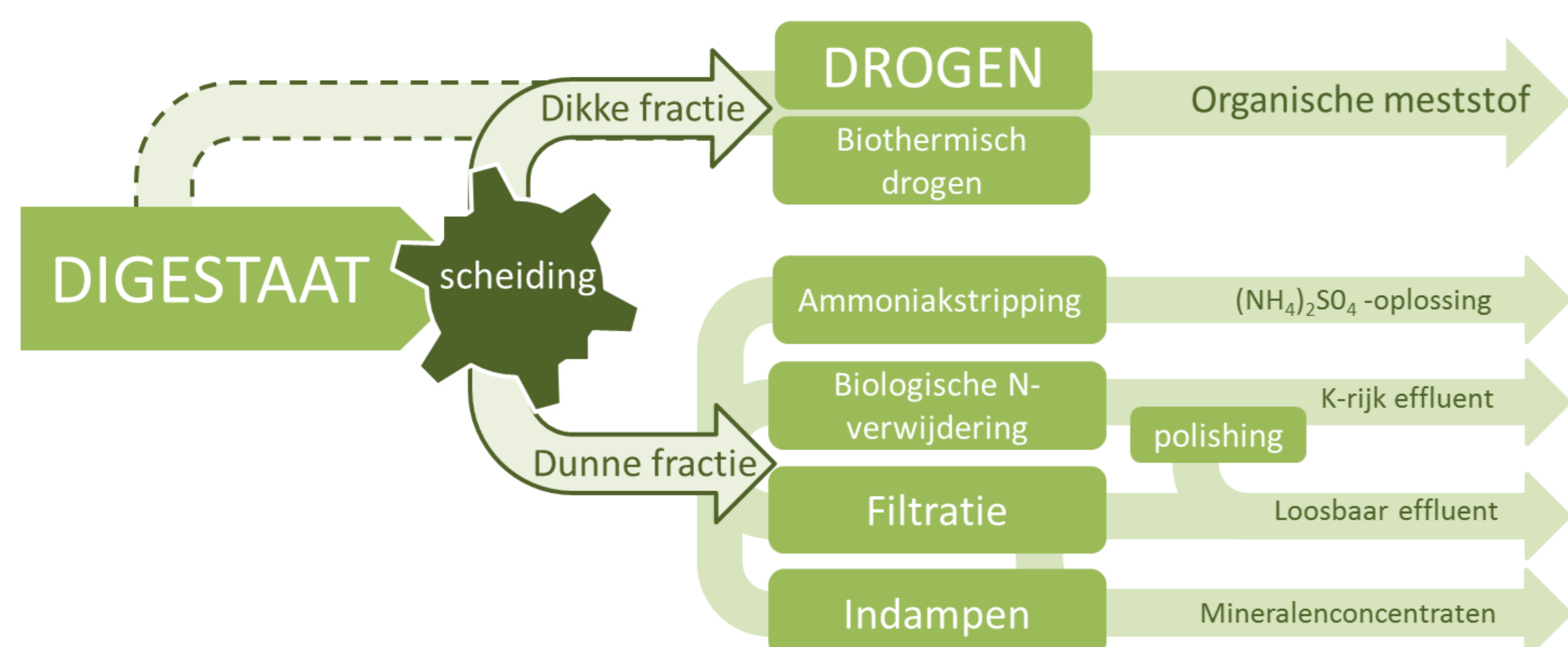
Figuur 2. Toegepaste nabehandelingstechnieken op digestaat van mest co-vergistingsinstallaties (bron: VCM-enquête 2010)
